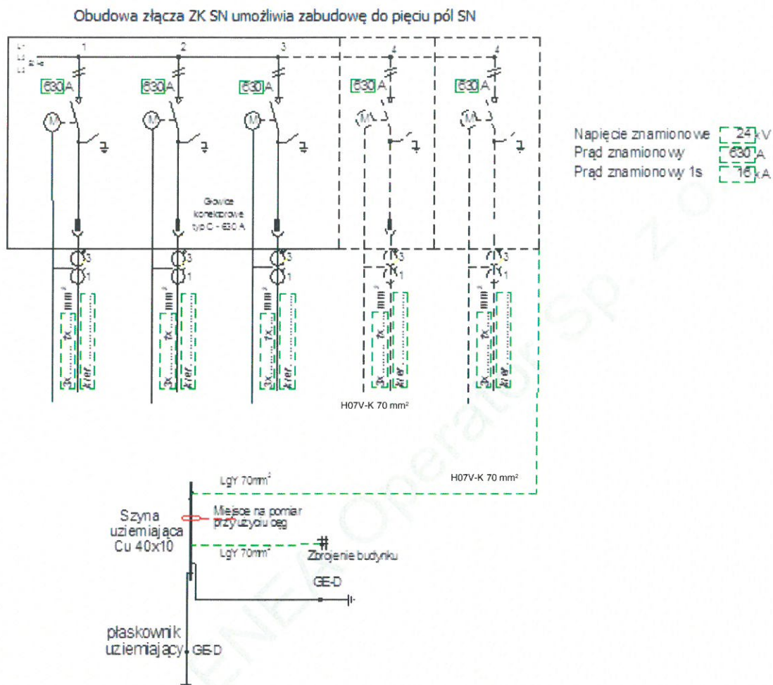
Rysunek nr 5a. Schemat złącza/szafy kablowej SN – wariant 1 – bez telemechaniki
