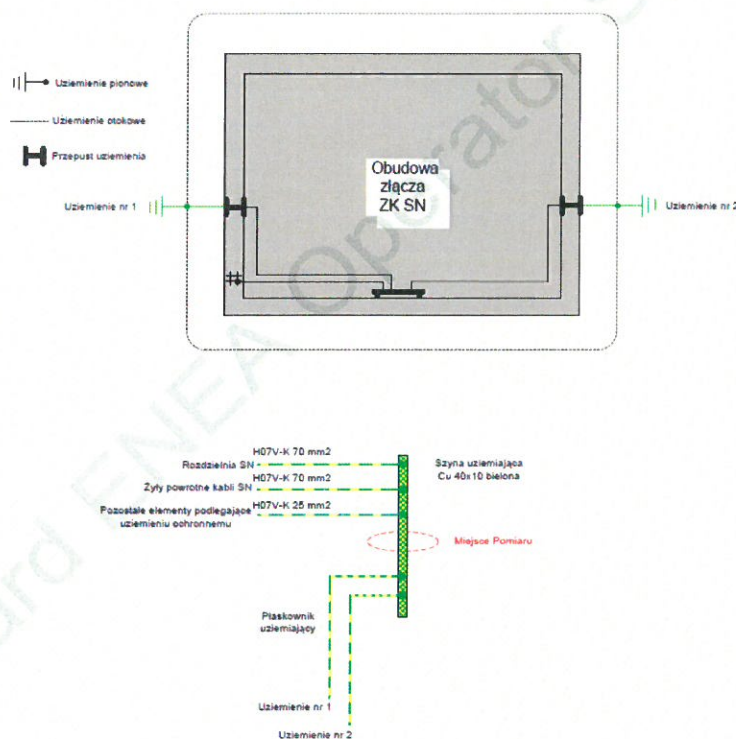
Rysunek nr 8. Uziemienie złącza/szafy kablowej SN
