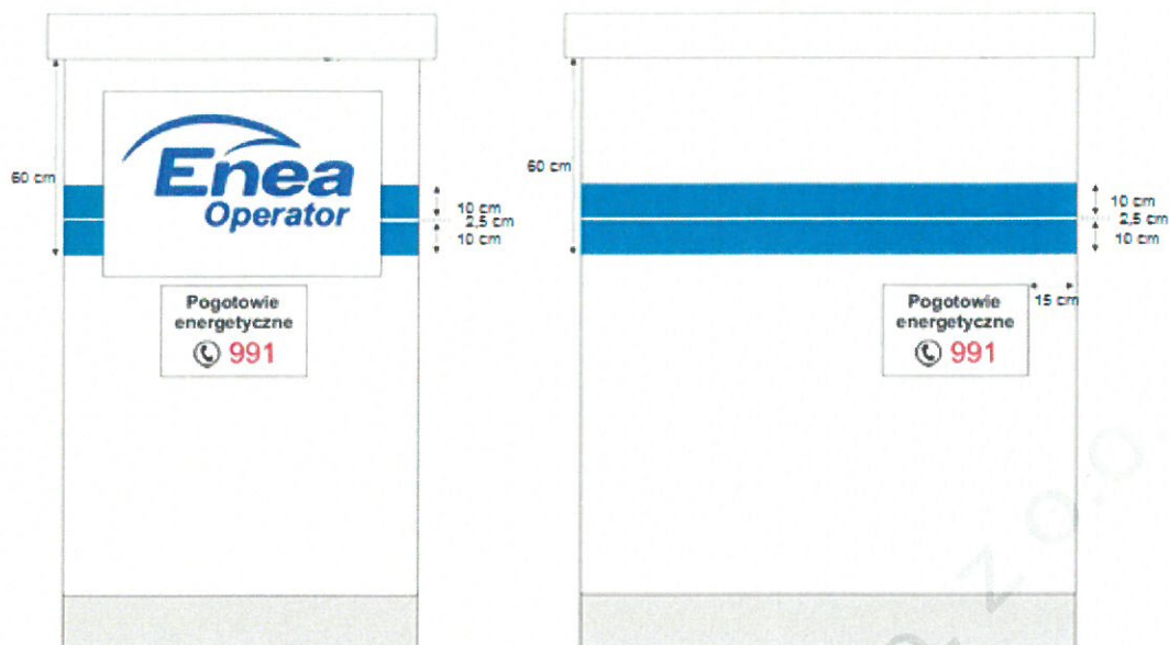
Rysunek nr 7. Wymiary oznakowania
