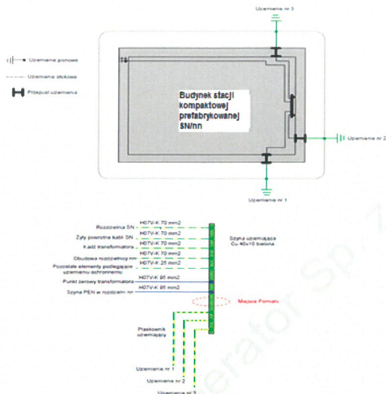
Rysunek nr 4. Uziemienie stacji SN/nn
