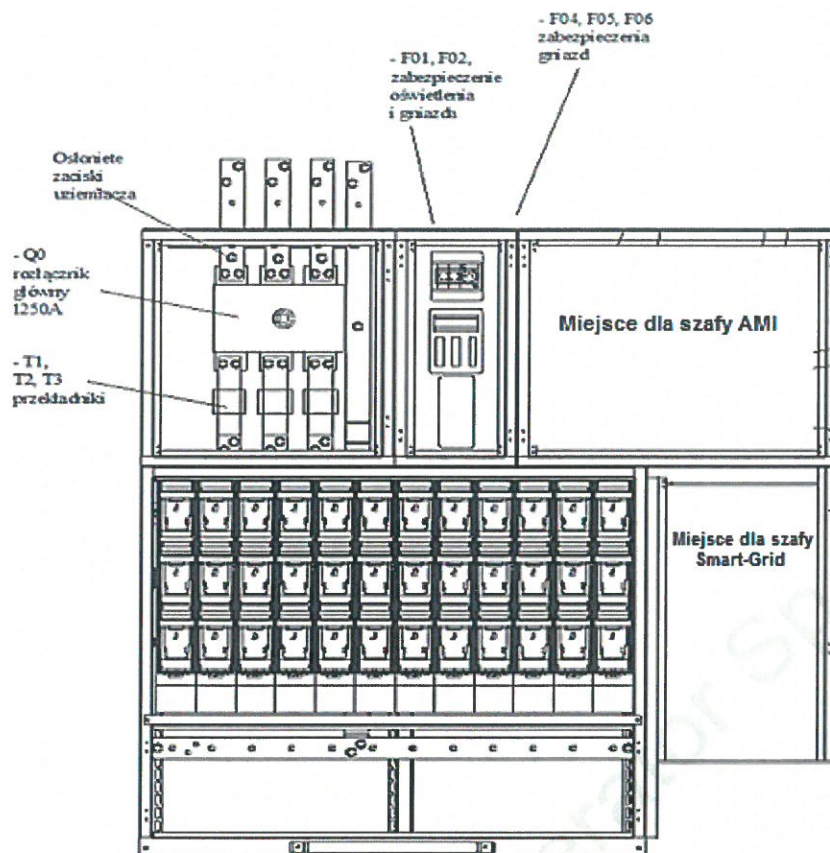
Rysunek nr 2. Rozmieszczenie elementów w rozdzielni nn (dopuszcza się wykonanie lustrzane)
